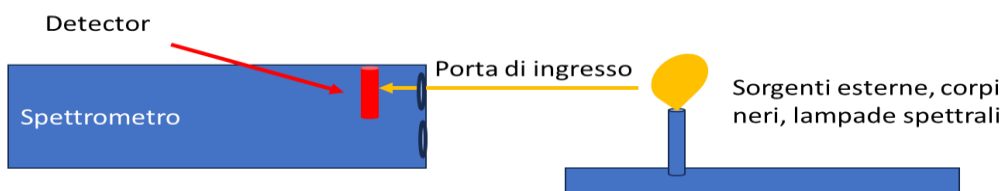
Figura 2: Configurazione per la caratterizzazione di sorgenti esterne
