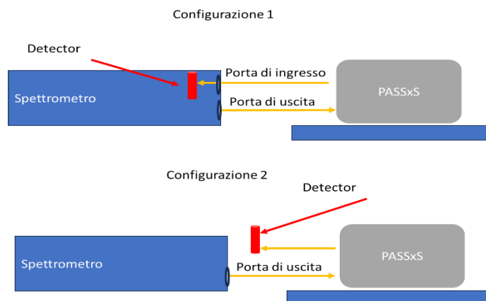
Figura 1: Configurazione 1 con detector interno (in alto) e configurazione 2 con detector esterno (in basso)
